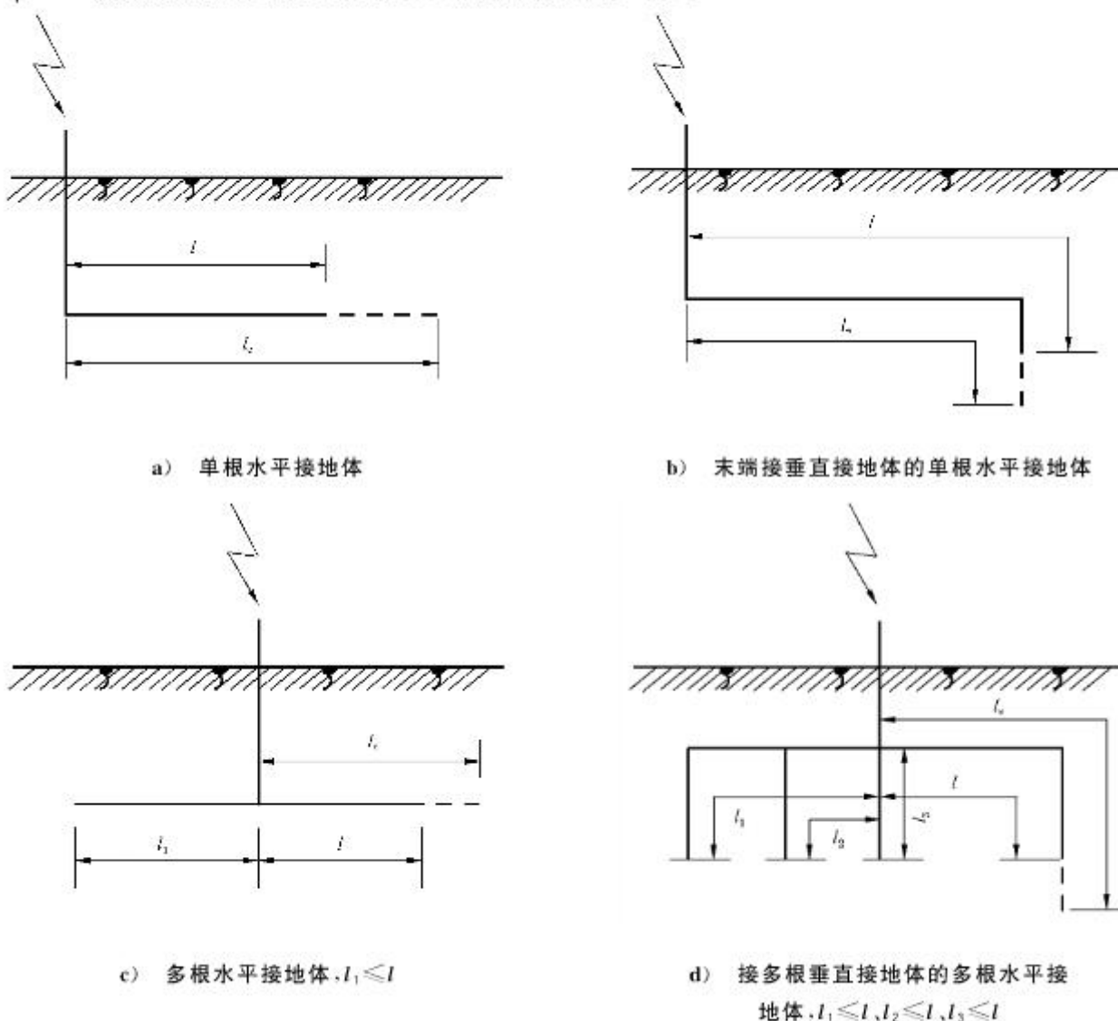
图 H.2 接地体的有效长度
