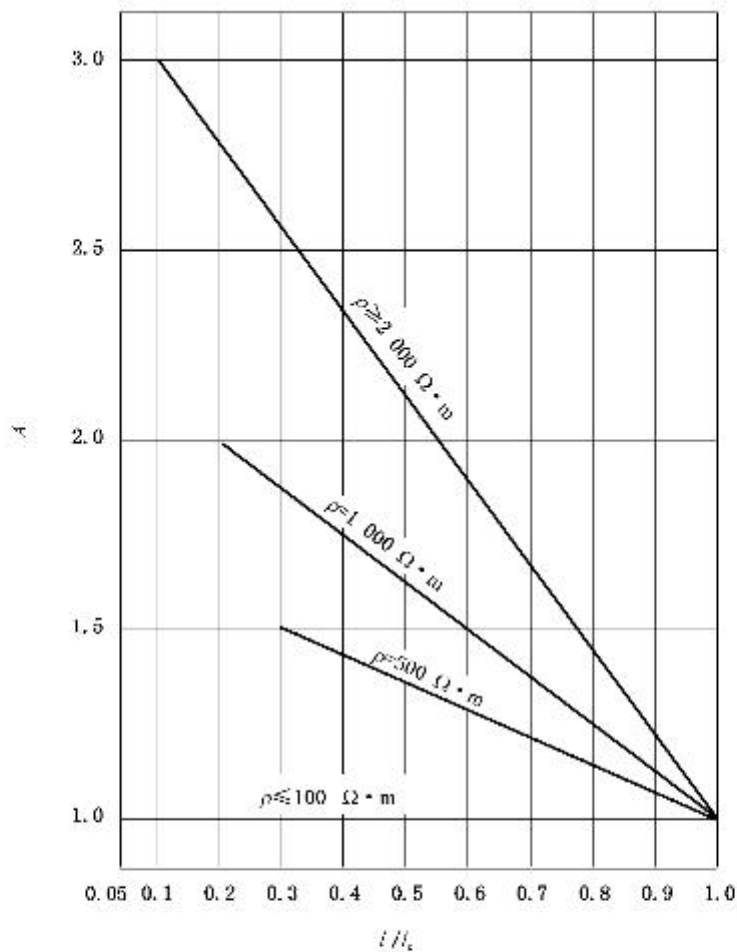
图 H.1 换算系数 A
